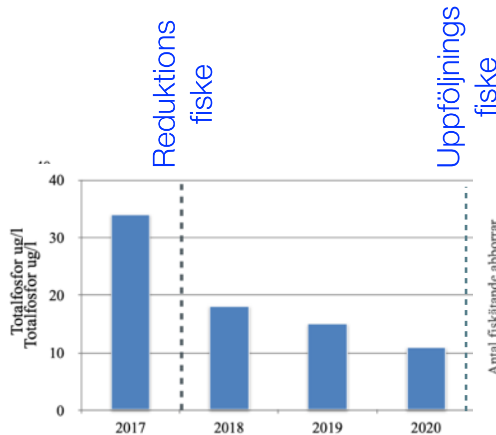
Totalfosfor (ug/l) i augusti i Sirsjön. Streckade linjen indikerar tidpunkt för reduktionsfiske.
